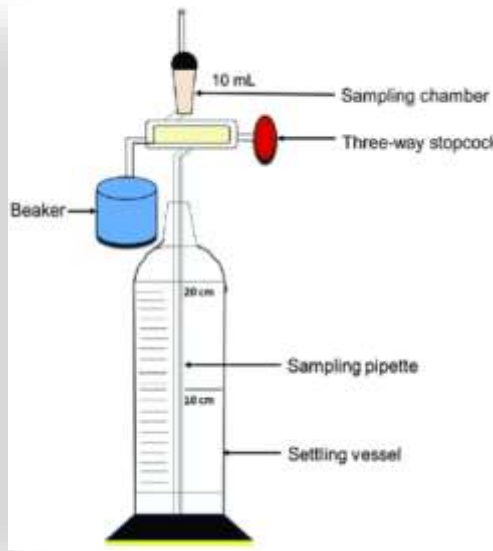
ANDREASEN APPARATUS
