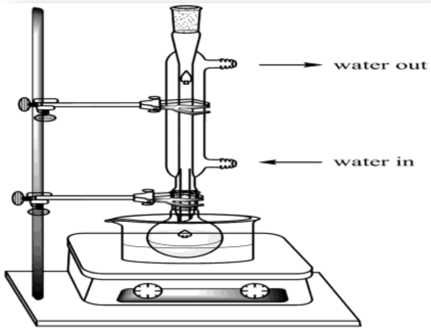
REFLUX
